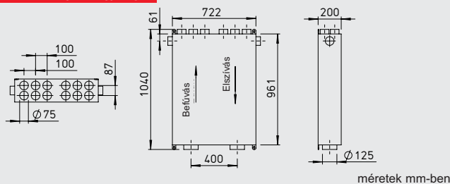
méretetek mm-ben
