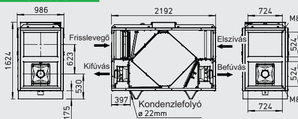
Méretetek mm-ben
