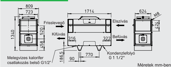
Melegvízes kalefifer csatlakozás belső G1/2"
