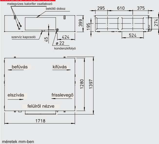
méretek mm-ben
