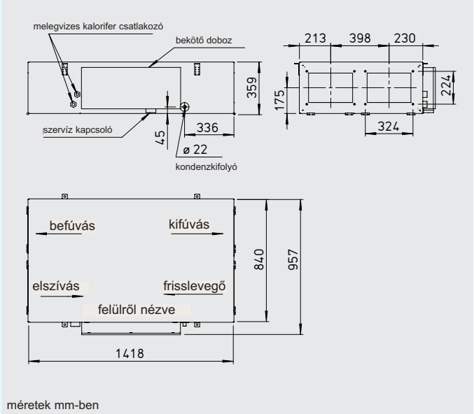
méretek mm-ben
