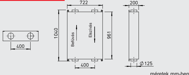
méretetek mm-ben
