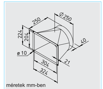
méretetek mm-ben
