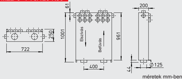
méretetek mm-ben
