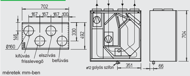
méretek mm-ben
