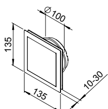
Méretetek mm-ben
