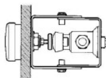
távműködtető különböző falvastagságokhoz ref. 18925 0,1 és 1,5 cm között ref. 18926 1,5 és 20 cm között ref. 18927 20 és 30 cm között ref. 18910 rögzítő keret
